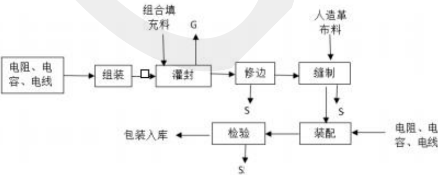
图 2-2 项目高铁配套产品生产工艺流程 G-废气 S-固废
