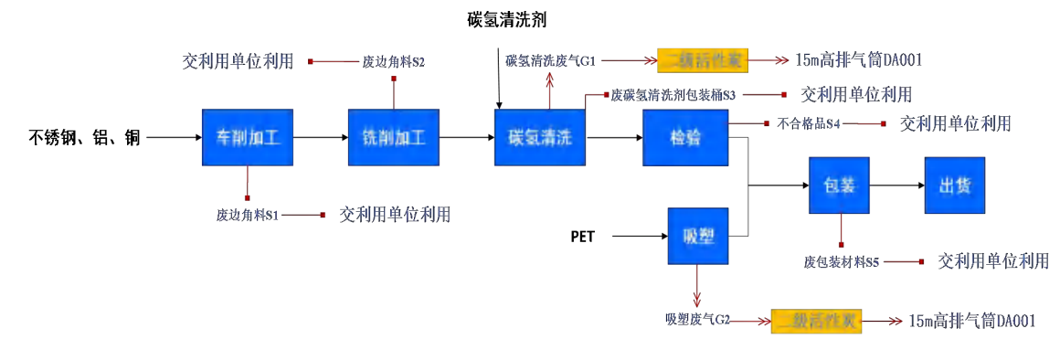
图 2-2 金属精密组件生产工艺流程图
