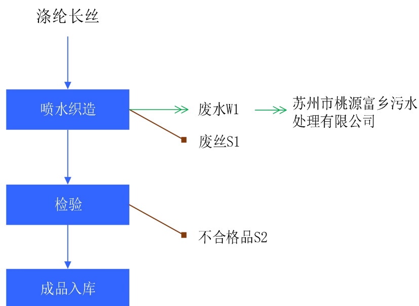
图 2-2 喷水织造生产工艺流程图
