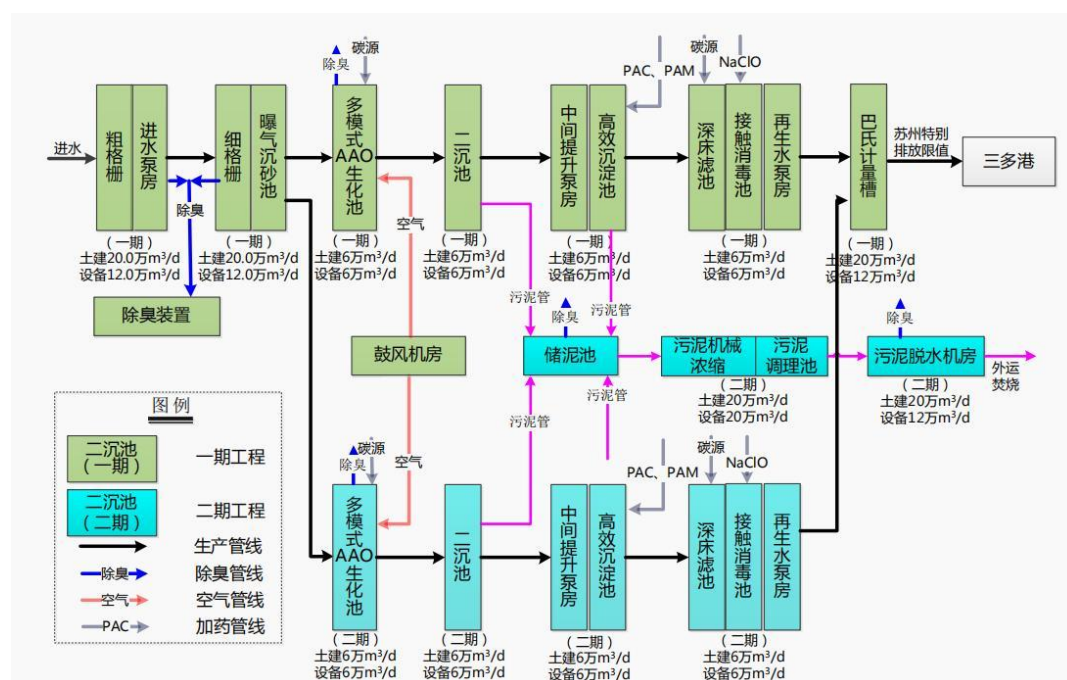
图 4-3 苏州市吴江城南污水处理有限公司工艺流程图
