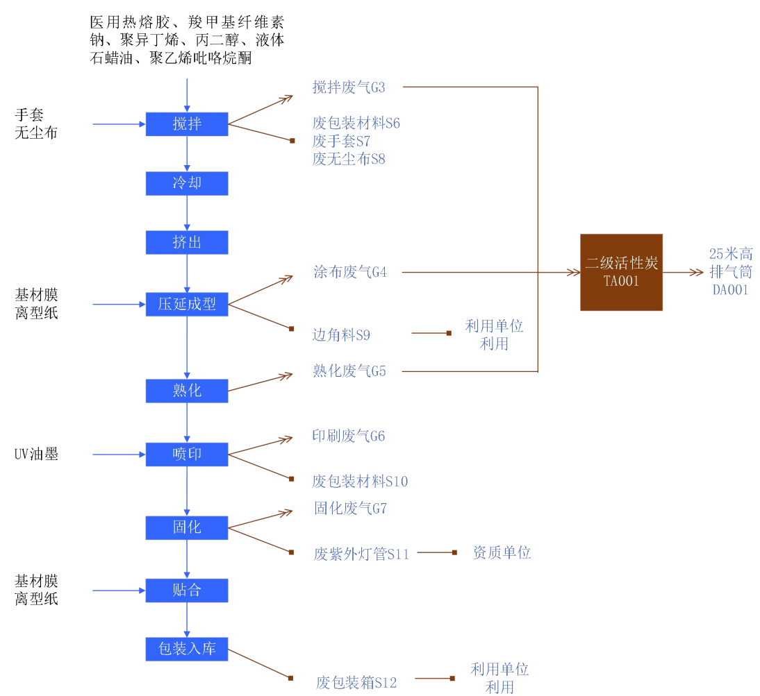
图 2-3 本项医用水胶体敷料生产工艺流程图
