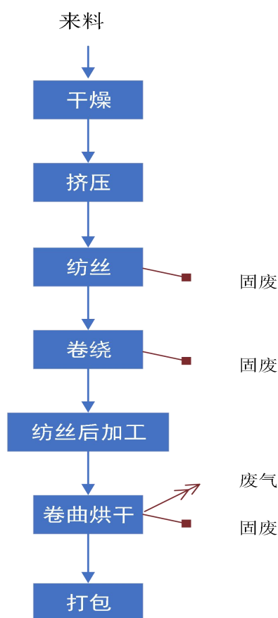
图 2-3 生产工艺流程图
