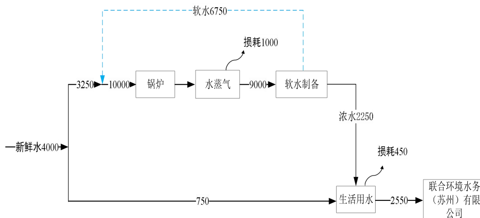
图 2-1 本项目全厂水平衡图 (t/a)
