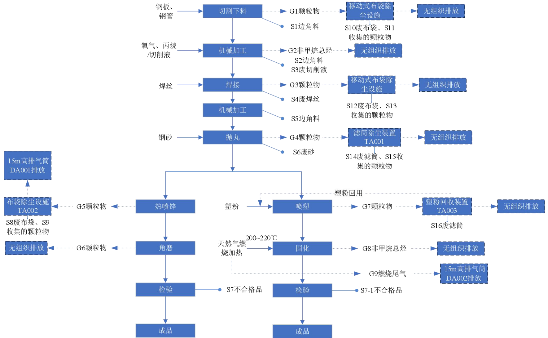
图 2-3 生产工艺流程图
