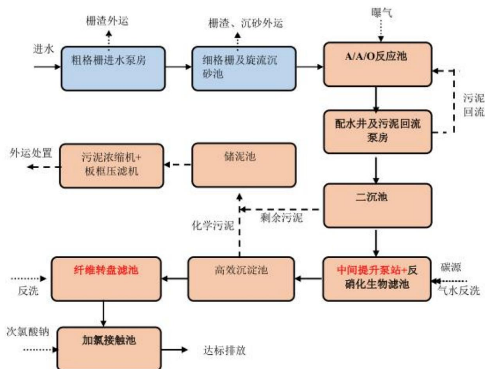
图 4-5 污水处理工艺流程图
