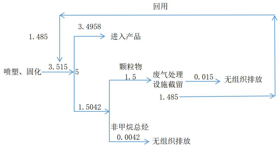
图 2-2 本项目塑粉平衡图 (t/a)
