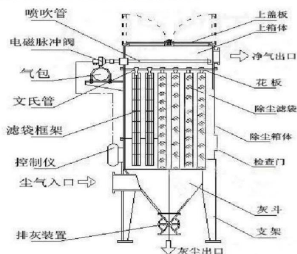
图 4-2 布袋除尘装置示意图
