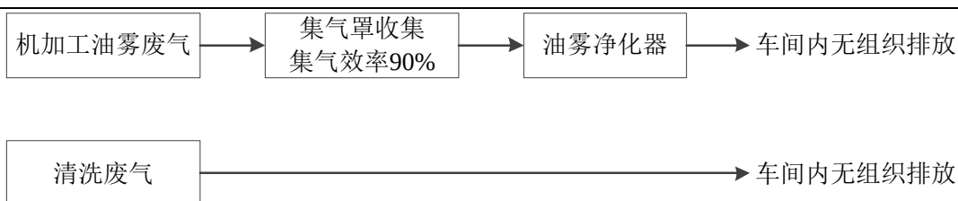
图 4-1 本项目废气处理流程图
