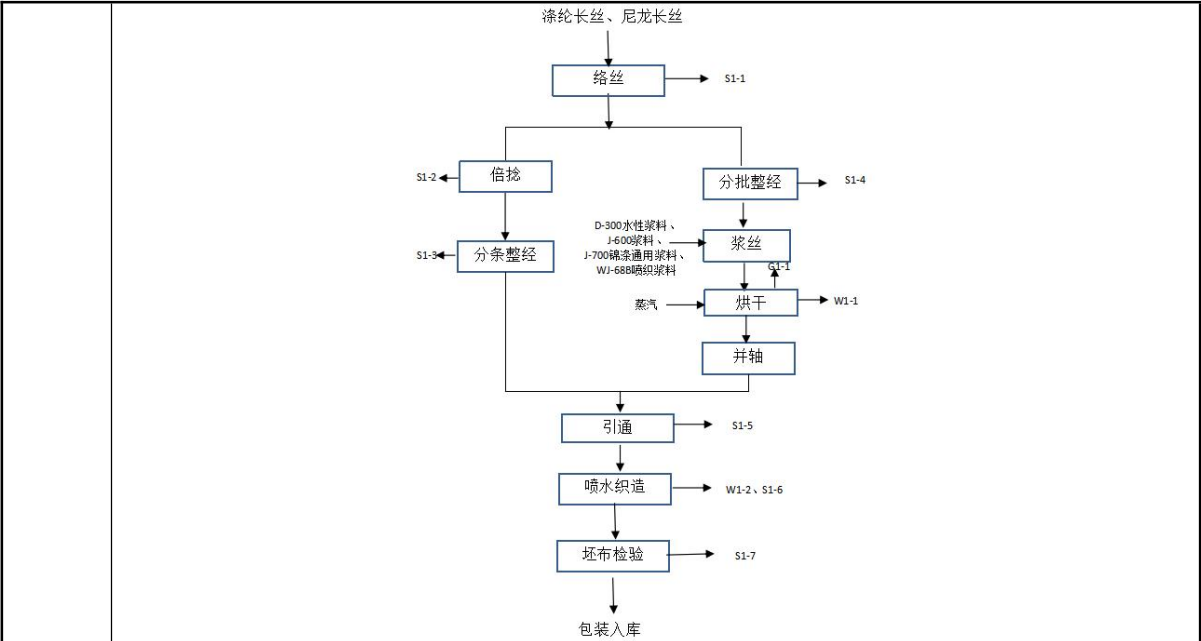
图 2-4 现有项目生产及产污环节示意图
