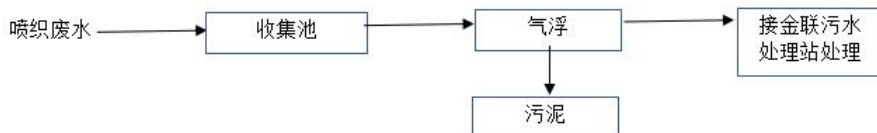
图 4-2 自建污水处理设施处理工艺流程
