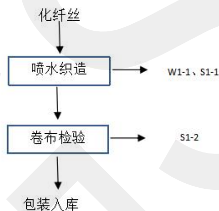
图 2-2 生产工艺流程及产污环节示意图 S-固废 W-废水
