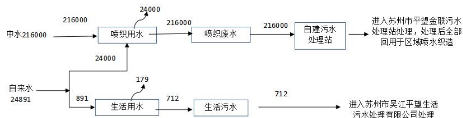
图2-1本项目水平衡图 t/a
