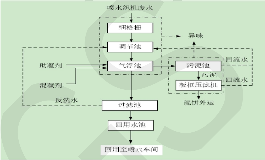
图 4-3 苏州市平望金联污水处理站处理工艺流程
