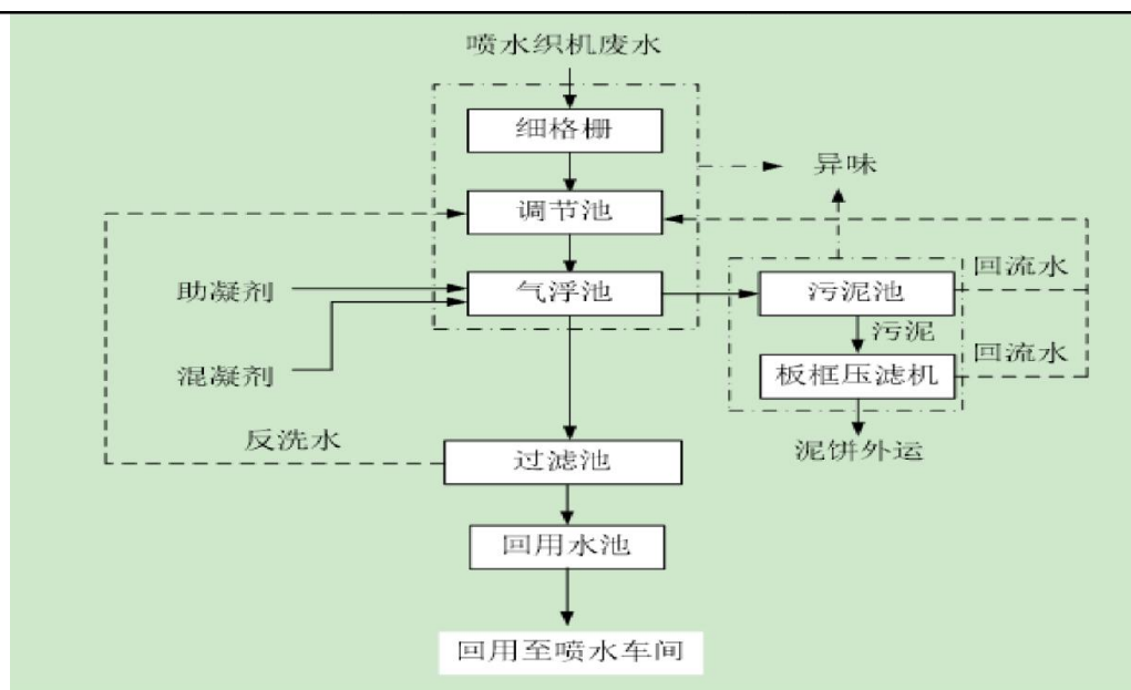
图 4-1 吴江市平望镇污水处理厂处理工艺流程
