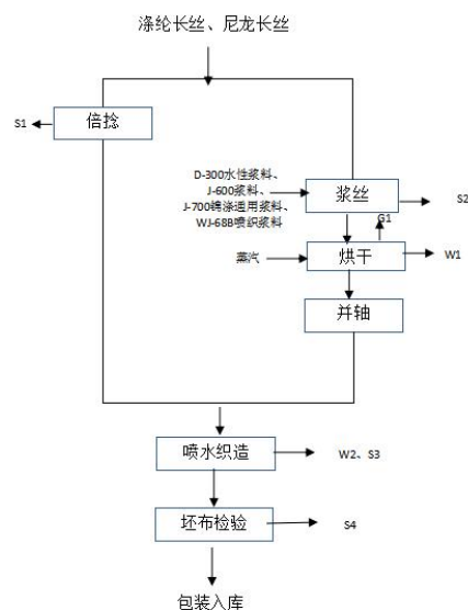
图 2-3 现有项目生产及产污环节示意图
