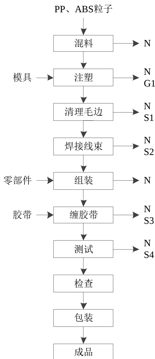
图 2-3 生产工艺流程图
