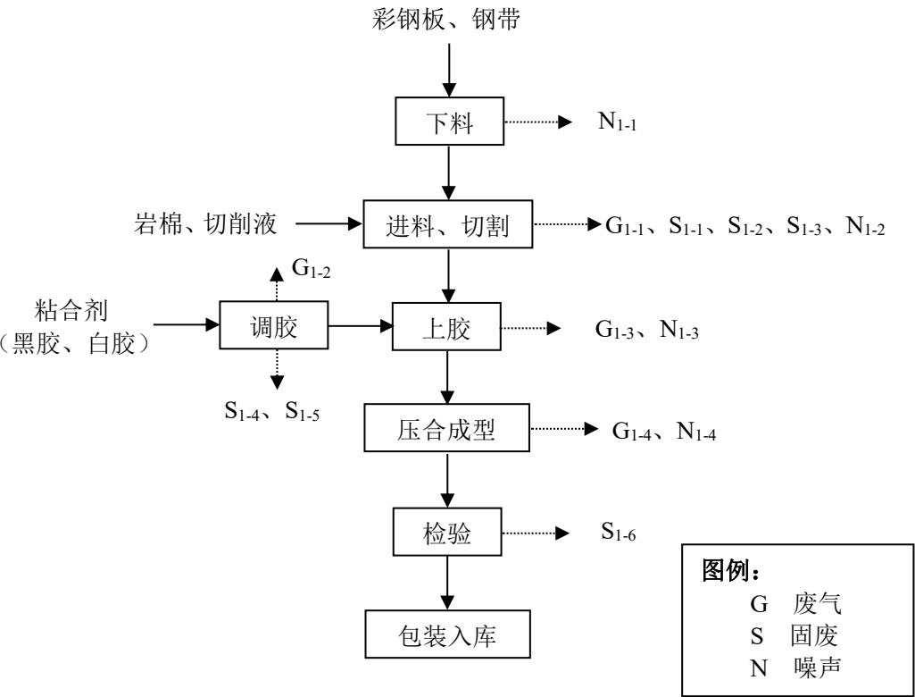
图 2-2 机制板工艺流程图
