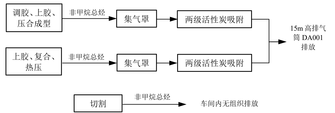
图 4-1 废气收集及处理方式图
