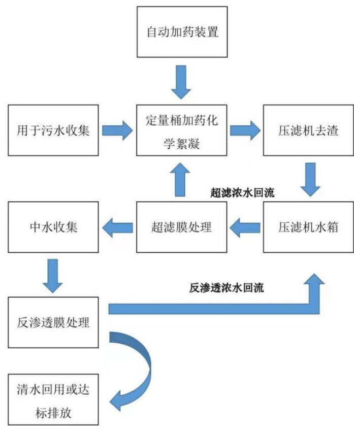
图 4-6 废水处理工艺流程图
