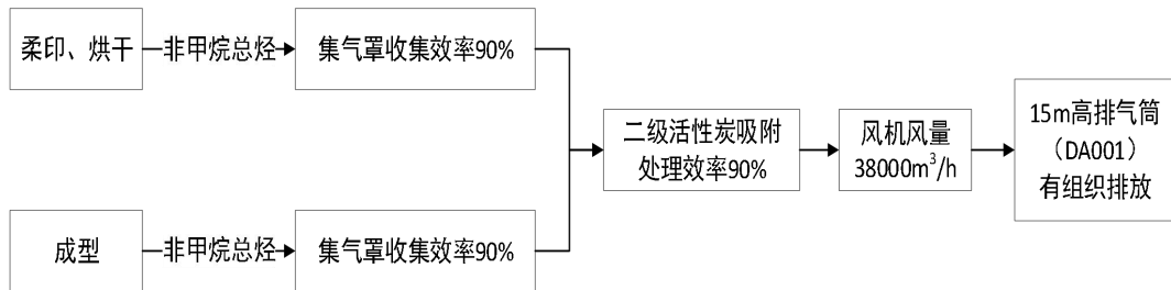
图 4-2 本项目废气处理流程图
