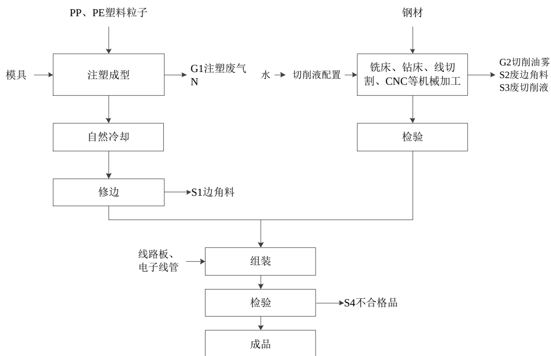
图 2-3 汽车零部件生产工艺流程图
