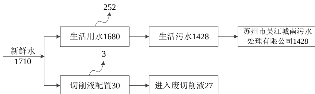
图 2-2 技改后全厂水平衡图 (t/a)
