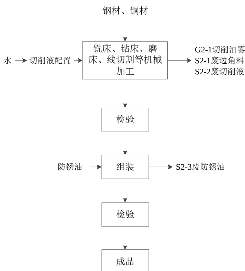
图 2-4 模具生产工艺流程图
