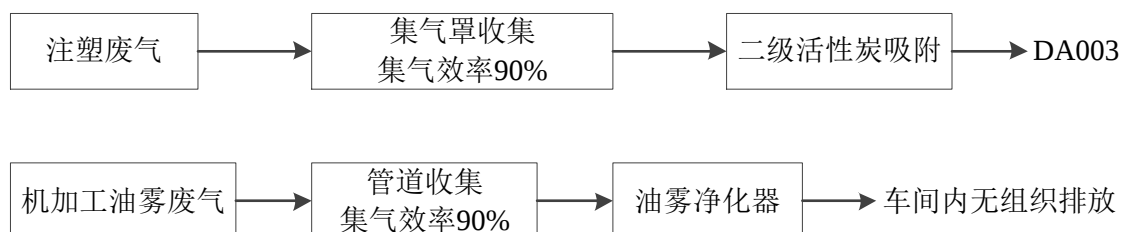
图 4-1 本项目废气处理流程图
