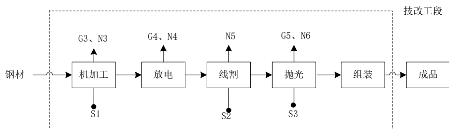
图 2-7 模具生产工艺流程图
