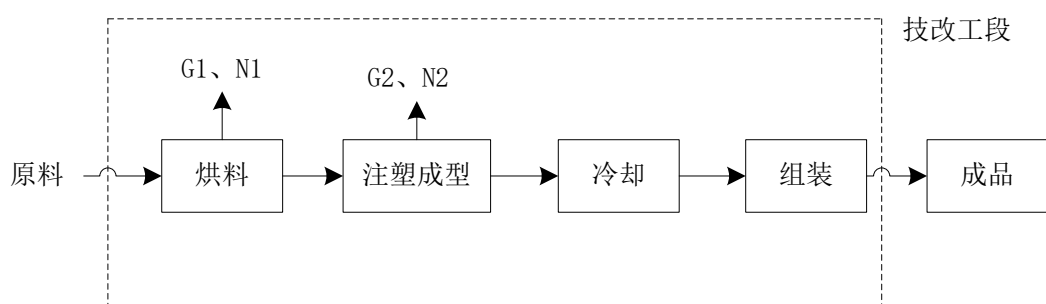
图 2-6 电子配件生产工艺流程图
