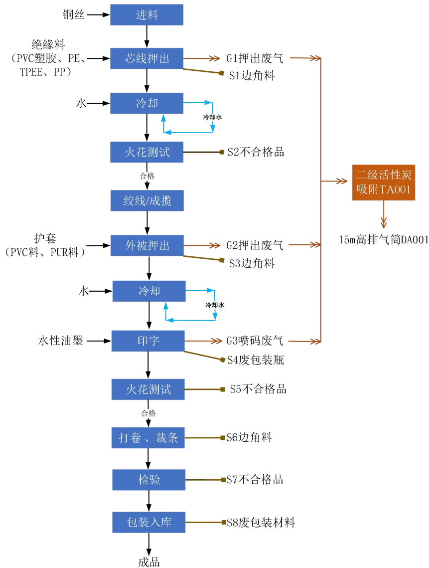
图 2-2 本项目生产工艺流程图
