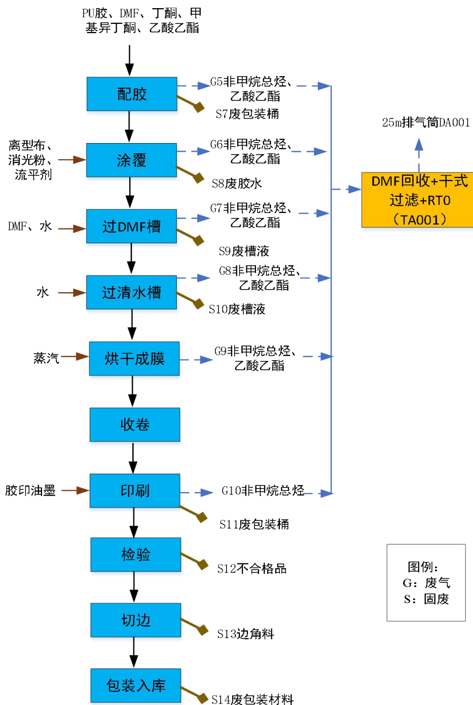
图2-3 微孔膜生产工艺流程及产污环节图
