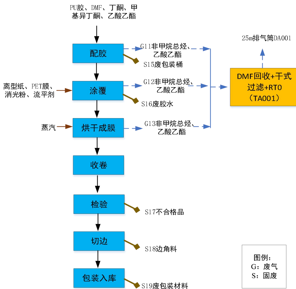
图2-4 多功能膜生产工艺流程及产污环节图
