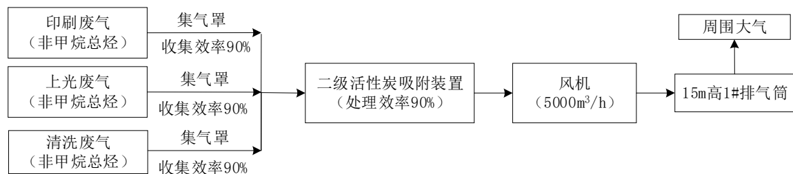
图 4-1 本项目废气收集处理图
