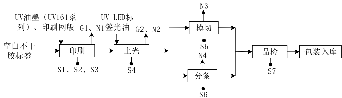
图 2-2 印刷不干胶标签工艺流程图
