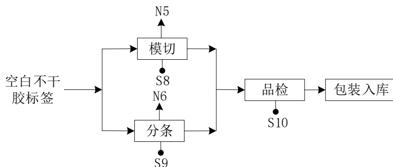
图 2-3 模切不干胶标签工艺流程图
