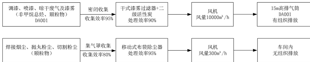
图 4-2 本项目废气处理流程图
