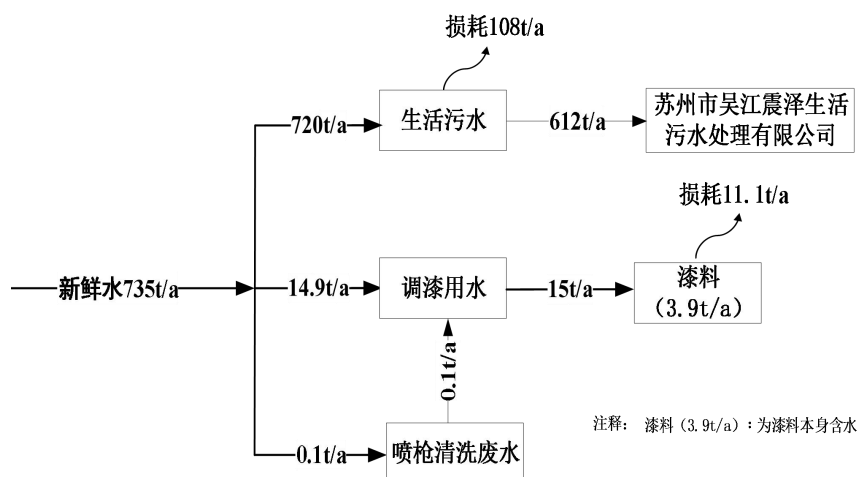
图 2-1 项目水平衡图 (t/a)
