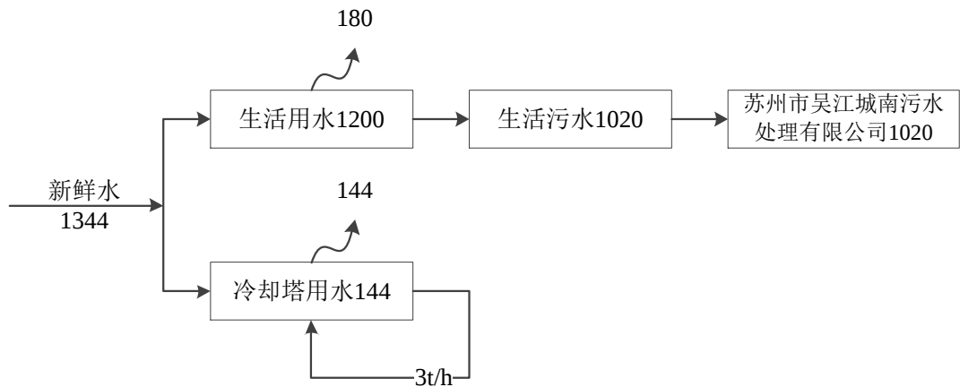
图 2-4 现有项目水平衡 (t/a)
