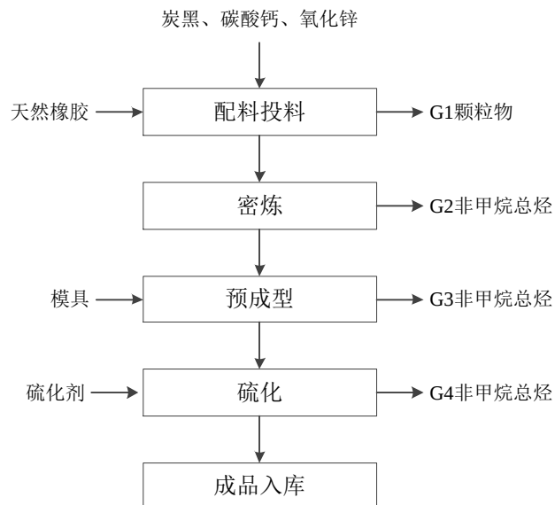
图 2-4 原有项目生产工艺流程图
