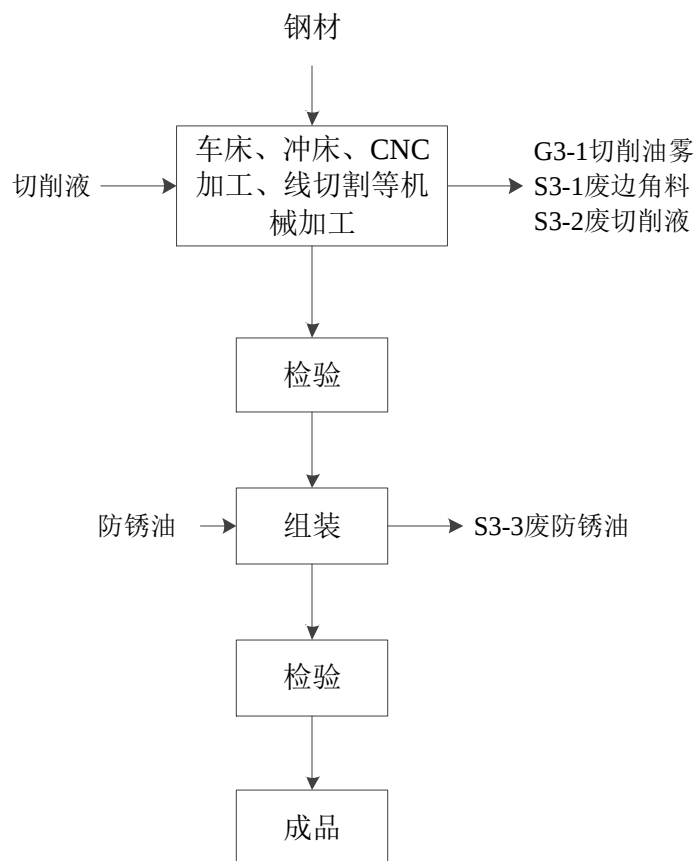
图 2-4 模具生产工艺流程图
