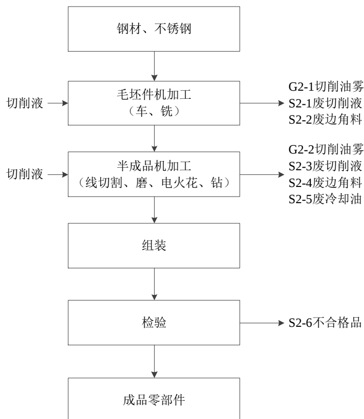
图 2-3 光伏零部件生产工艺流程图
