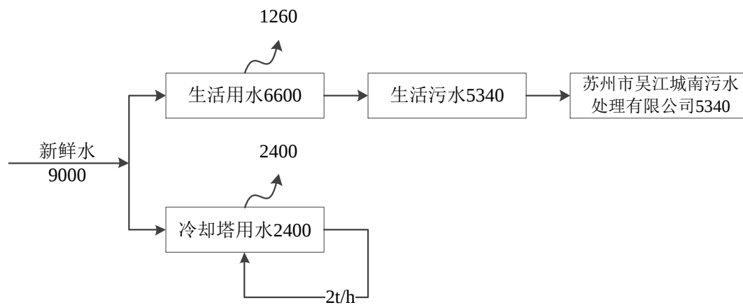
图 2-2 技改后全厂水平衡图 (t/a)
