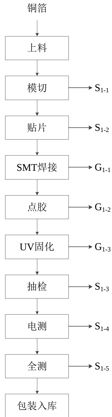
图 2-1 电子元器件生产工艺流程图
