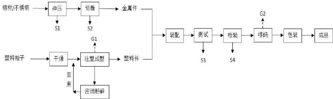
图 2-5 生产工艺流程图
