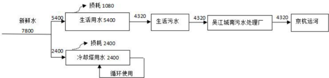
图 2-4 现有项目水平衡 (t/a)
