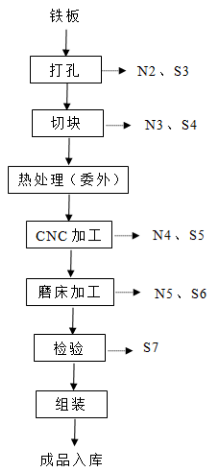
图 2-6 五金配件生产工艺流程图
