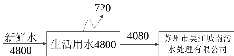
图 2-1 本项目水平衡图（t/a）
