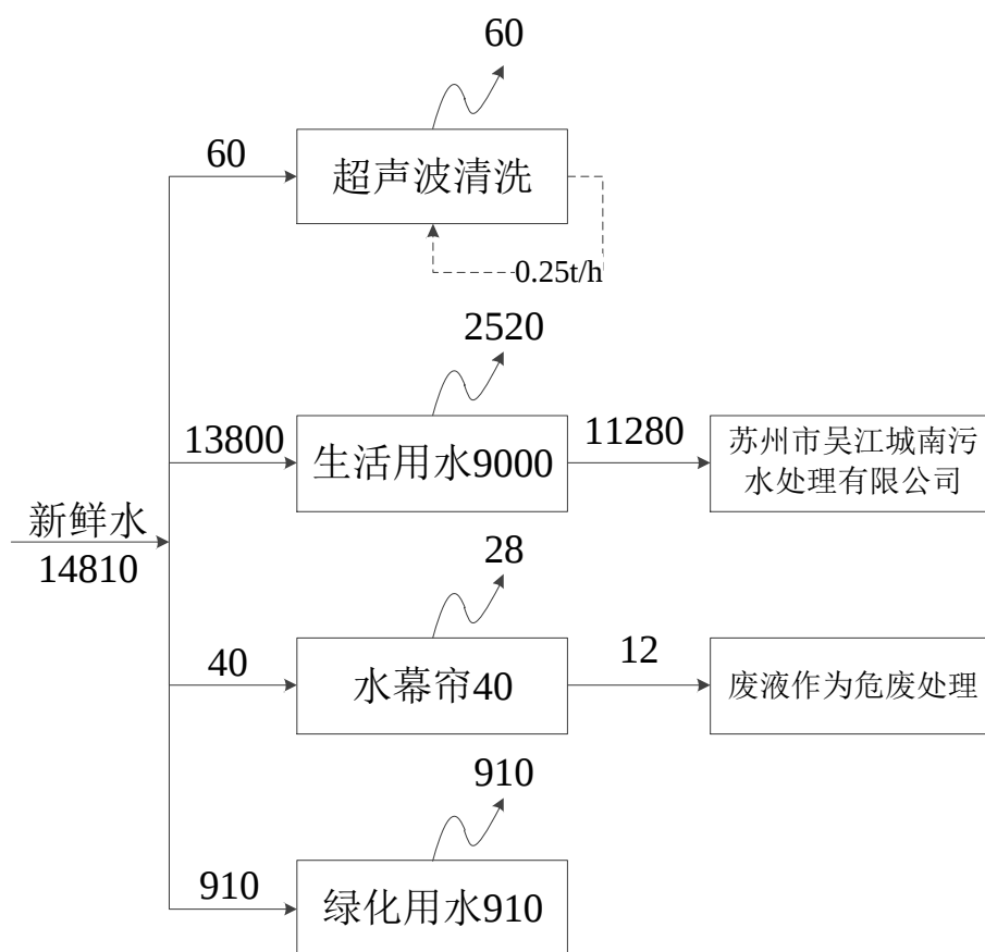
图 2-2 全厂水平衡图（t/a）
