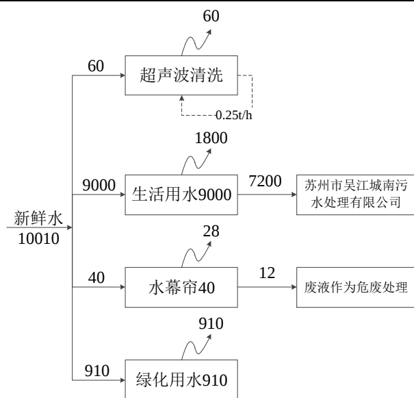
图 2-4 现有项目水平衡 (t/a)
