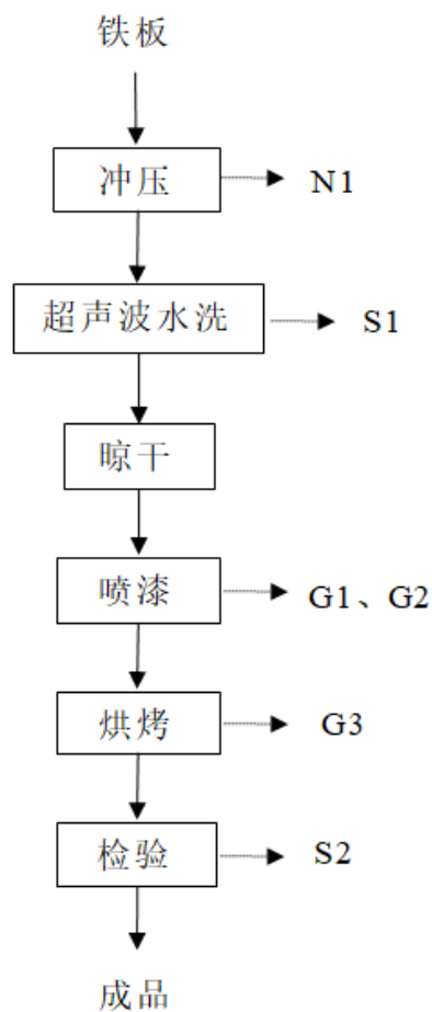
图 2-5 精密冲压件生产工艺流程图
