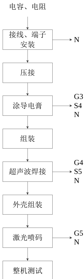
图 2-3 隔离开关生产工艺流程及产污环节图
