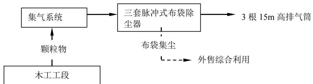
图 4-2 颗粒物处理工艺示意图
