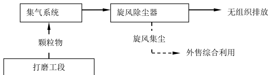
图 4-5 颗粒物处理工艺示意图
