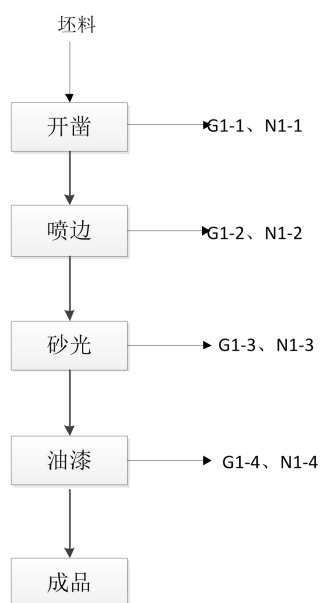
图 2-1 地板生产工艺流程图
