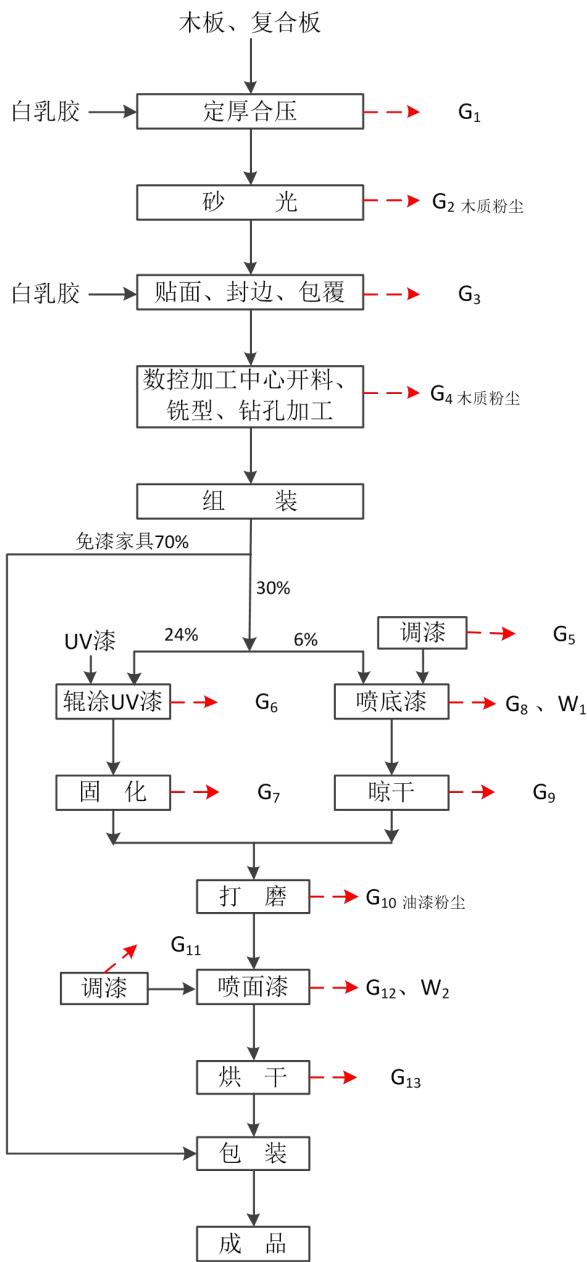
图 2-2 成套家具制造生产工艺流程图
