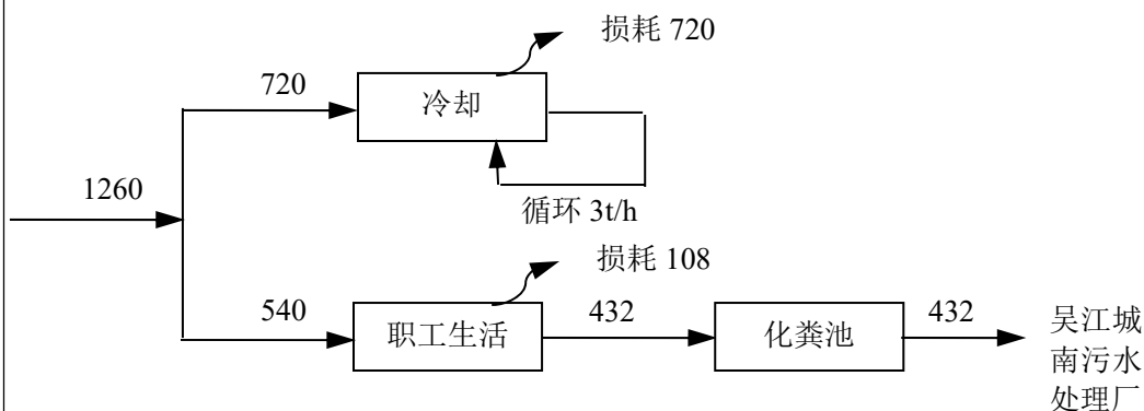
图 2-1 本项目水平衡图（单位：m³/a）
