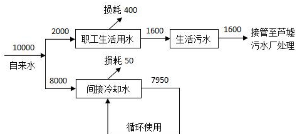
图 4-1 全厂水平衡图
