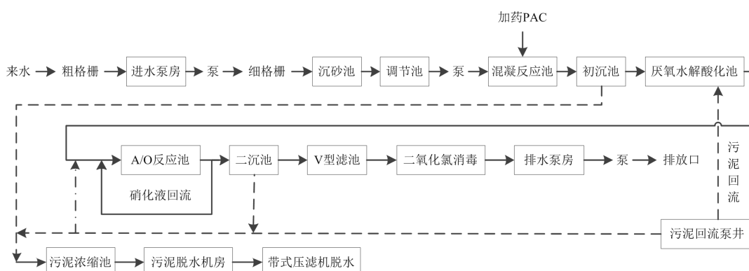
图 4-2 苏州市吴江区芦墟污水处理有限公司污水处理工艺流程图
