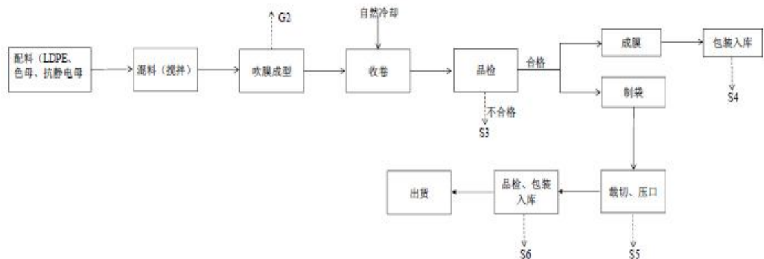
图 2-2 药用低密度聚乙烯膜（袋）生产工艺流程图
