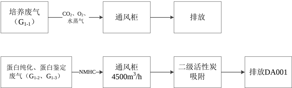
图 4-1 本项目集气方案图
