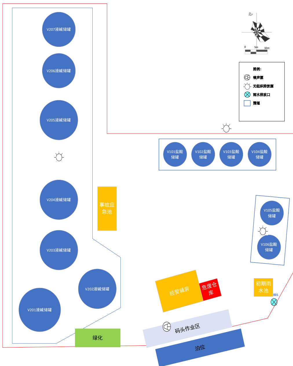
图 3-3 项目平面布置示意图
