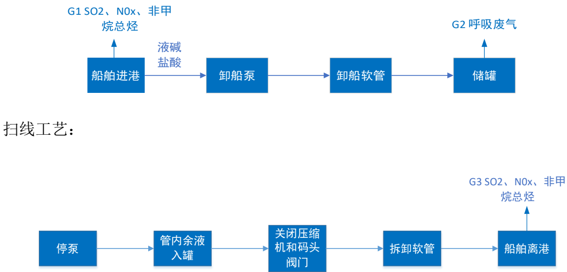
附图 3-5 工艺流程图
