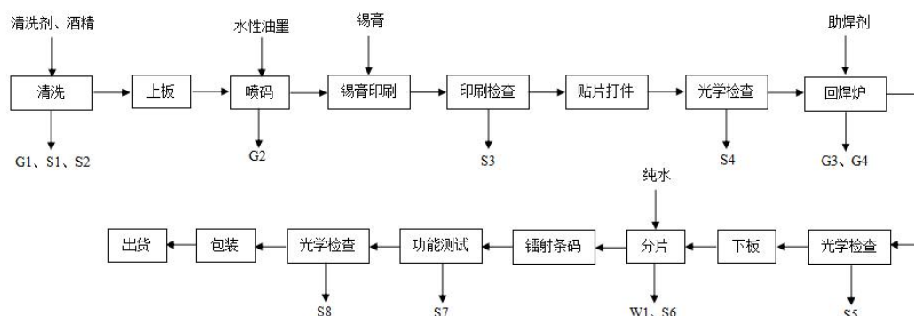
图 2-2 射频模块生产工艺流程图
