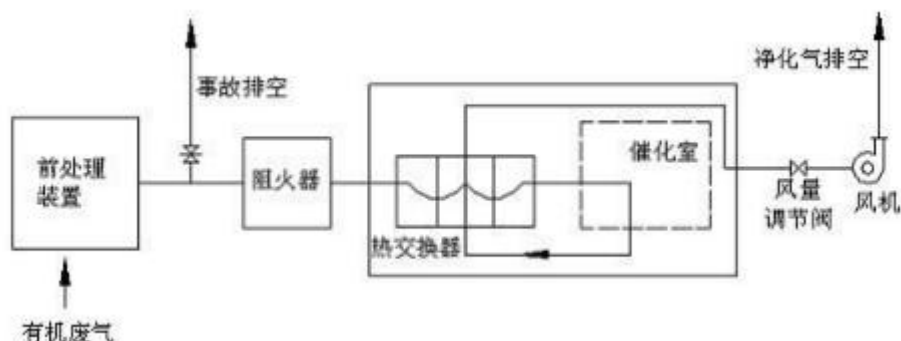
图 4-2 催化燃烧装置工作原理图
