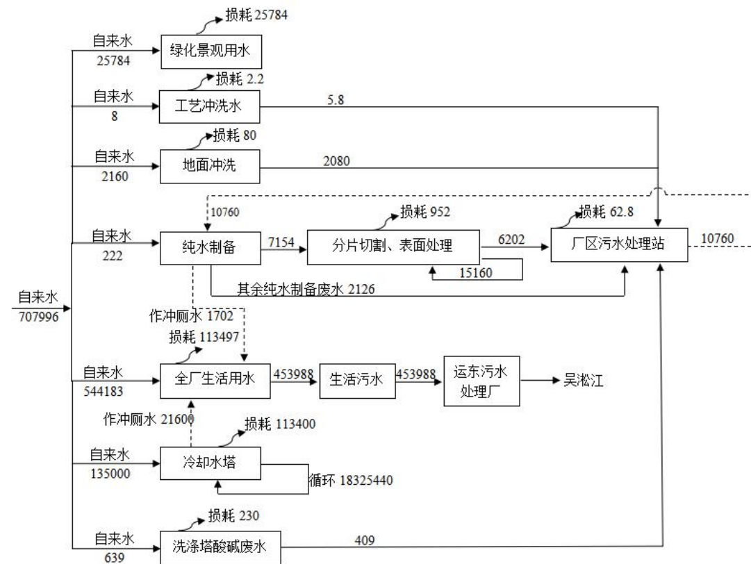
图 2-2 全厂水平衡图 (t/a)
