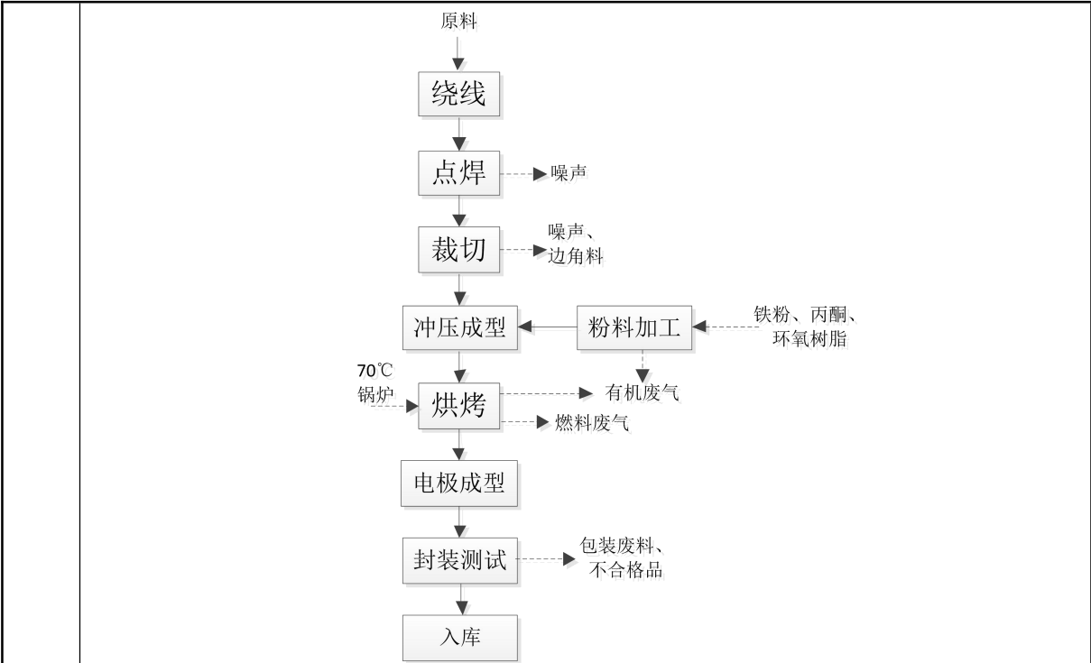
图 2-12 电子元器件工艺流程图
