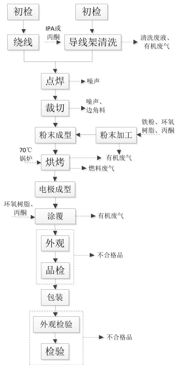
图 2-7 大电感生产线工艺流程
