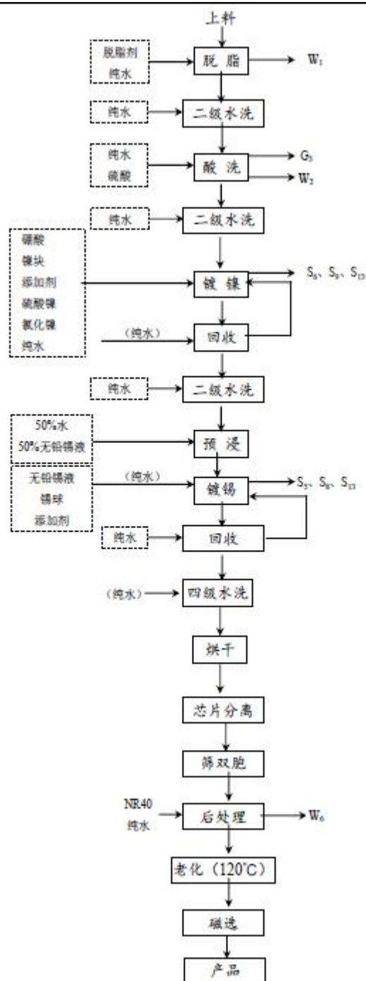
图 2-11 表面处理工艺流程图
