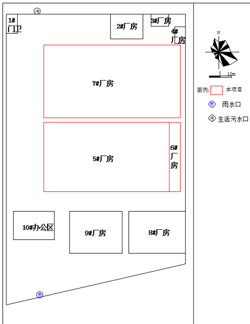
附图7 出租方厂区总平面布置图
