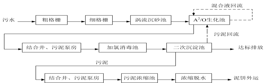
图 4-1 污水处理厂处理工艺流程图
