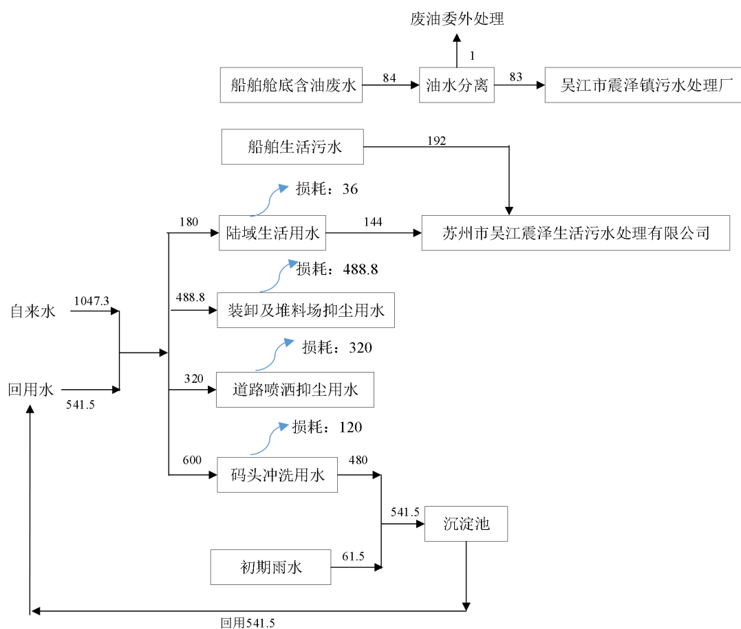
图 5-2 项目水平衡图
