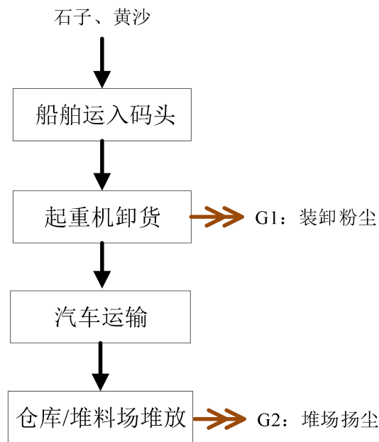
图 5-1 工艺流程图
