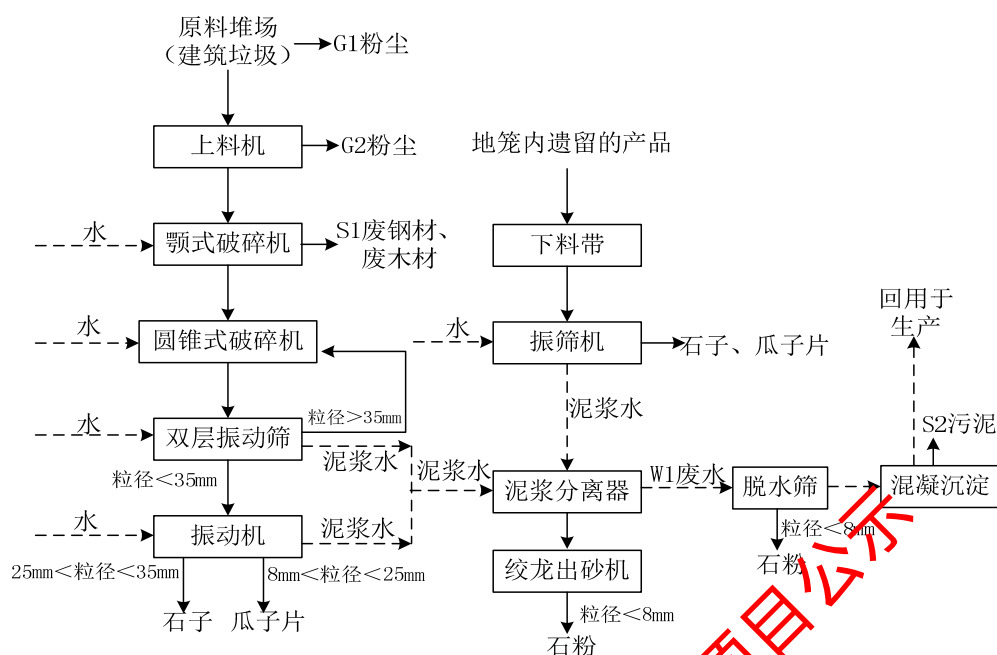
图 1-1 再生骨料生产工艺流程
