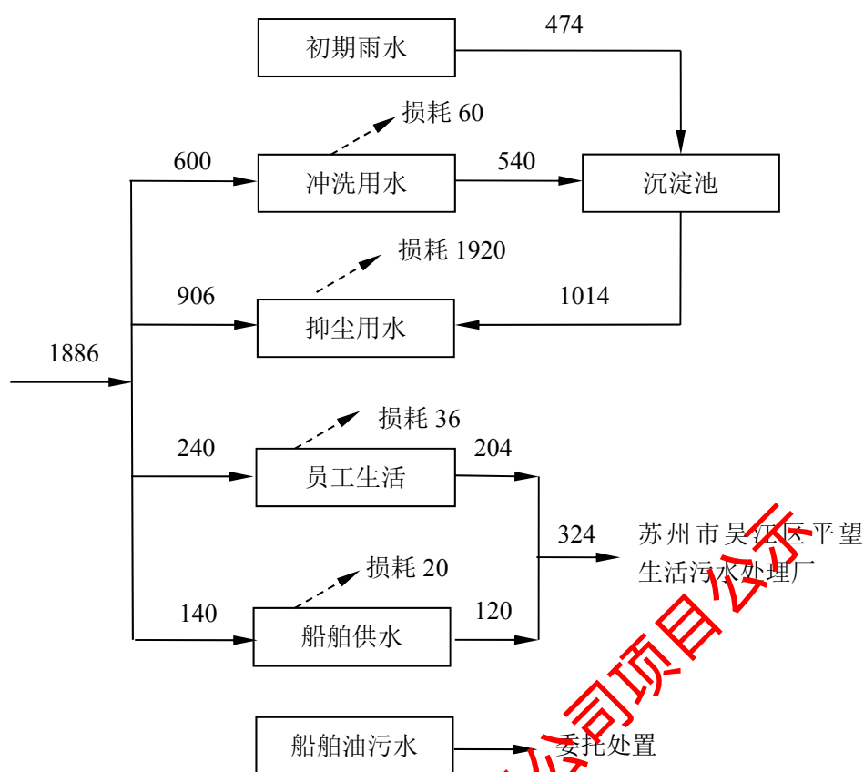
图 5-2 本项目厂区水平衡图 单位: m³/a
