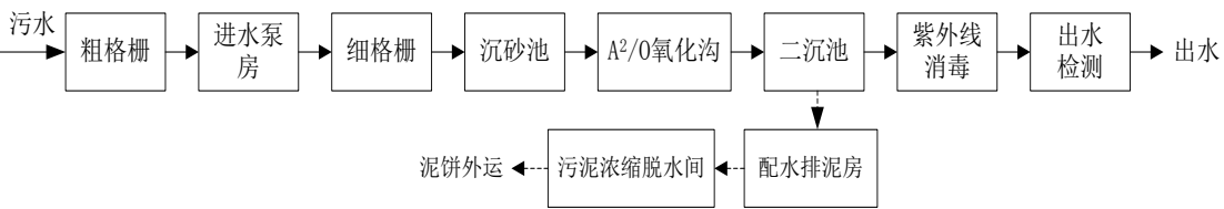
图 7-1 污水处理厂处理工艺图
