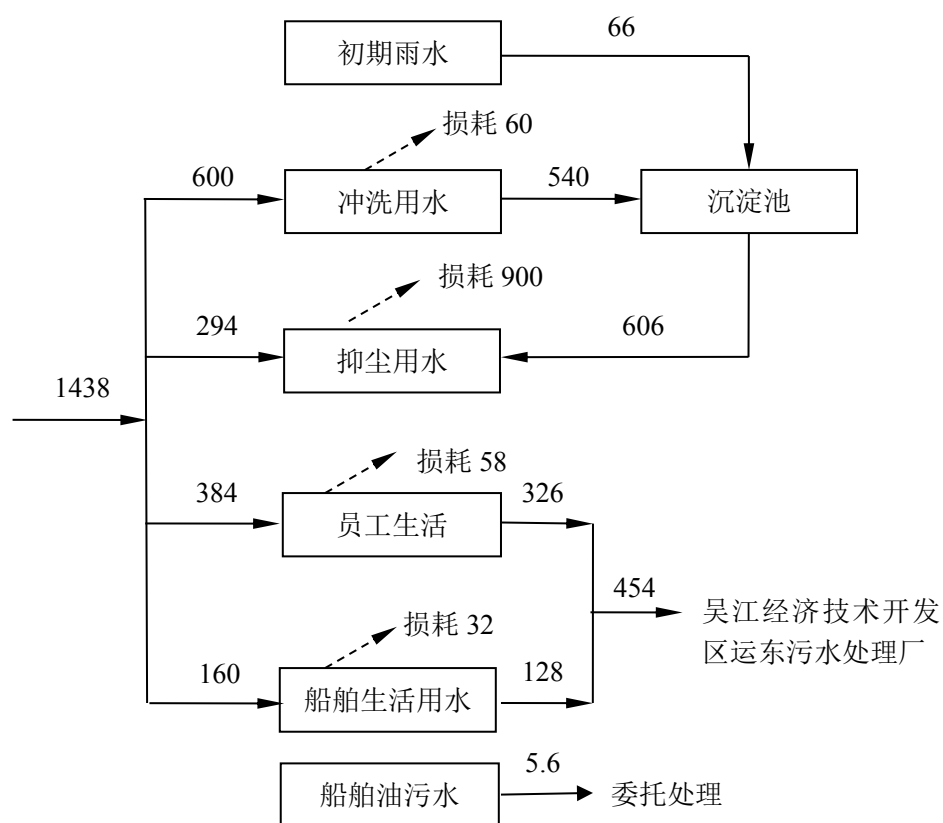
图 5-3 本项目厂区水平衡图 单位：m 3 /a
