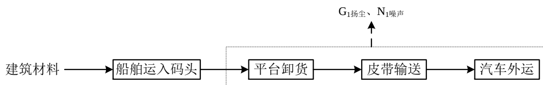
图 5-2 码头装卸工艺流程及产污环节示意图
