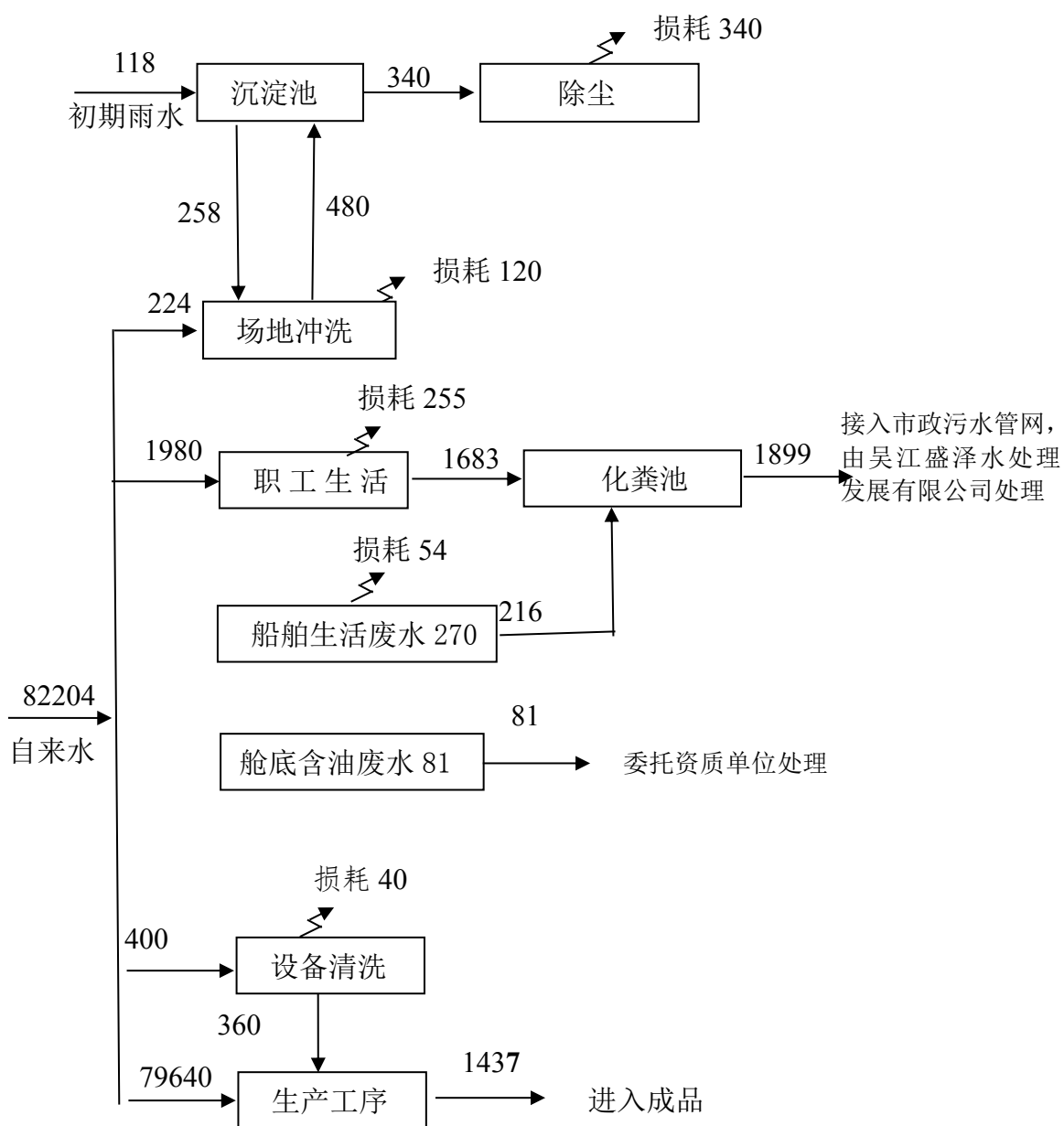
图 5-3 全厂用排水平衡图 (单位 t/a)
