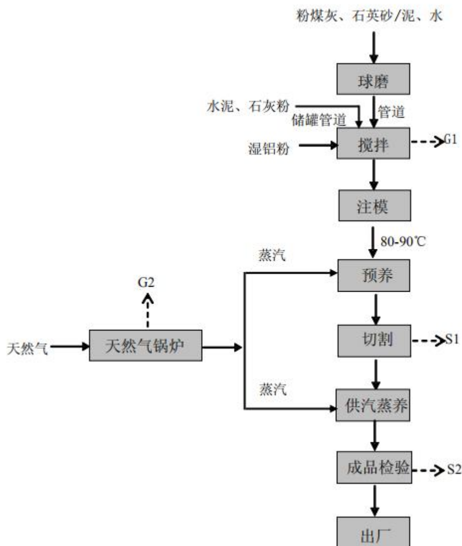
图 1-1 现有项目生产工艺流程图
