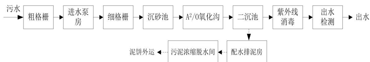
图 7-1 吴江区运东污水处理厂污水处理工艺流程图
