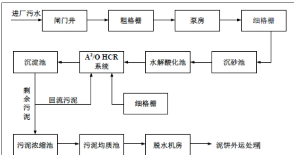
图 7-2 吴江市震泽镇污水处理厂处理工艺流程图
