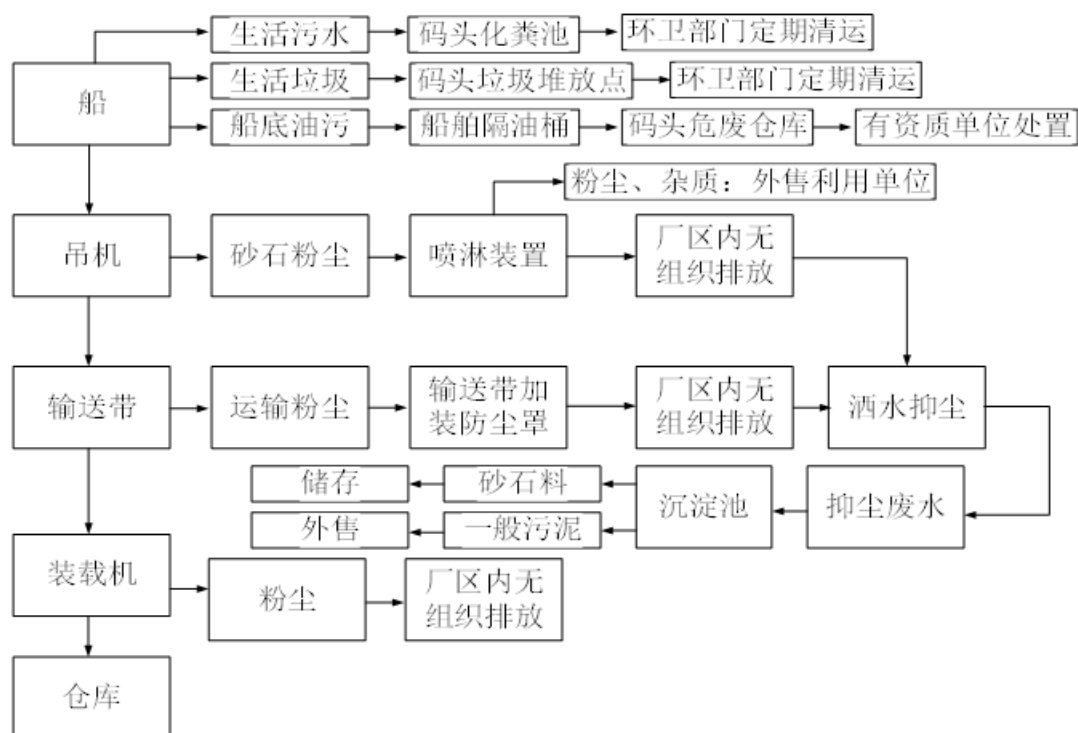
本项目装卸方案一
