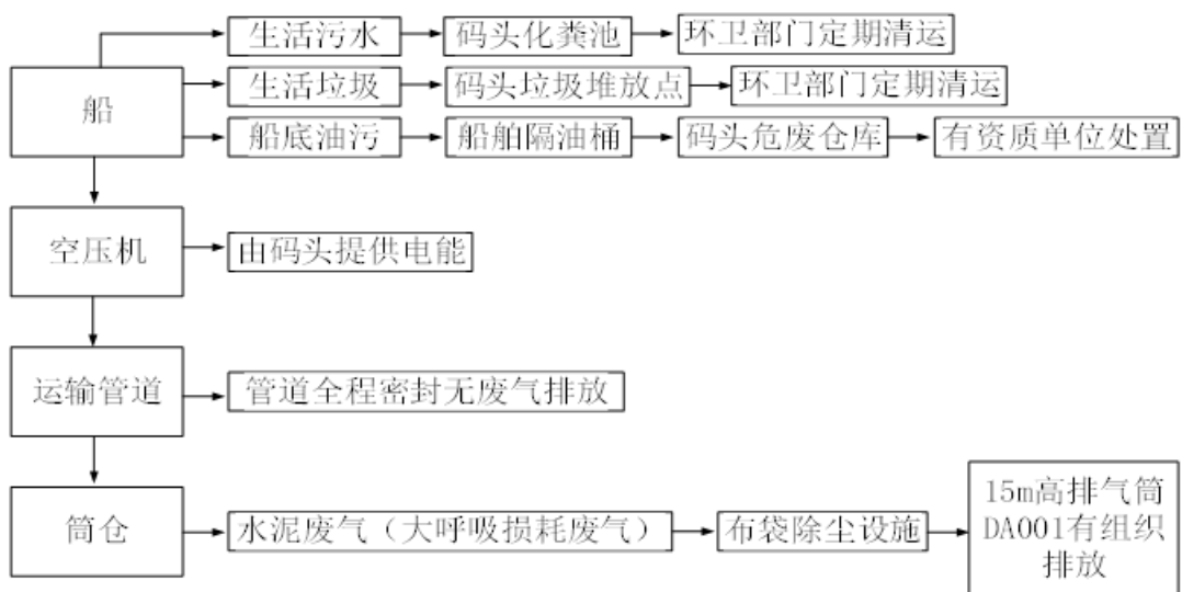
本项目装卸方案二
