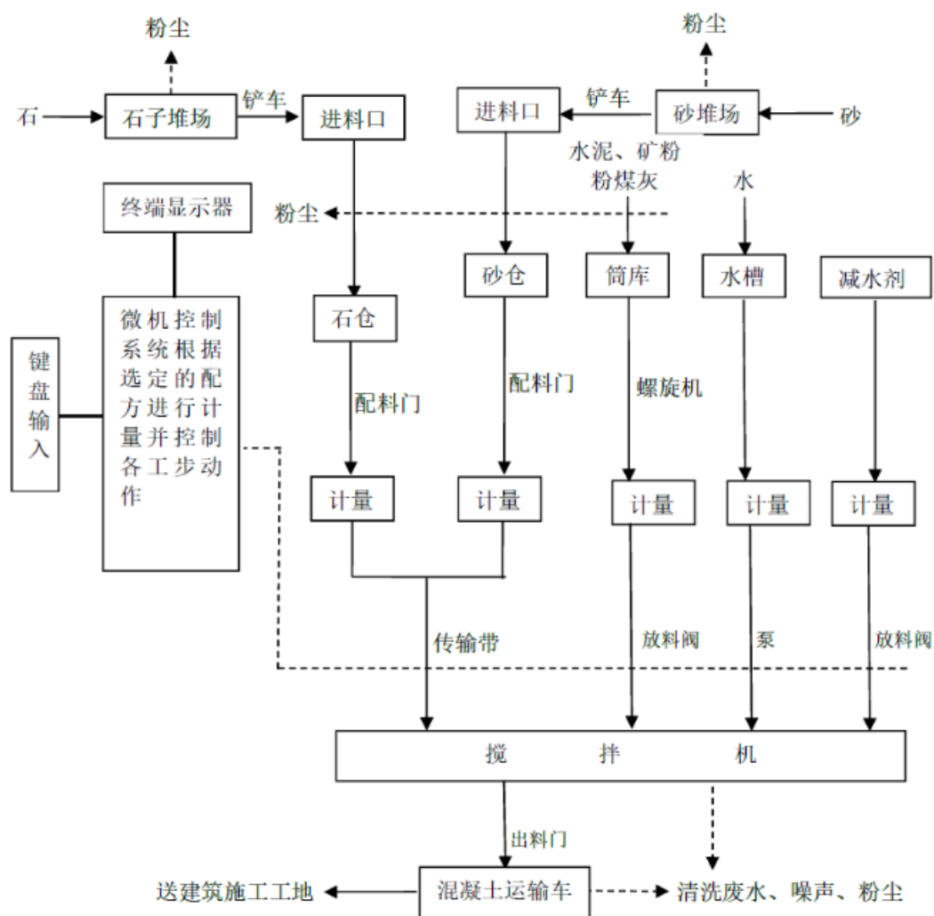
图 1-1 搬迁及“绿色生产”技术改造项目工艺流程图
