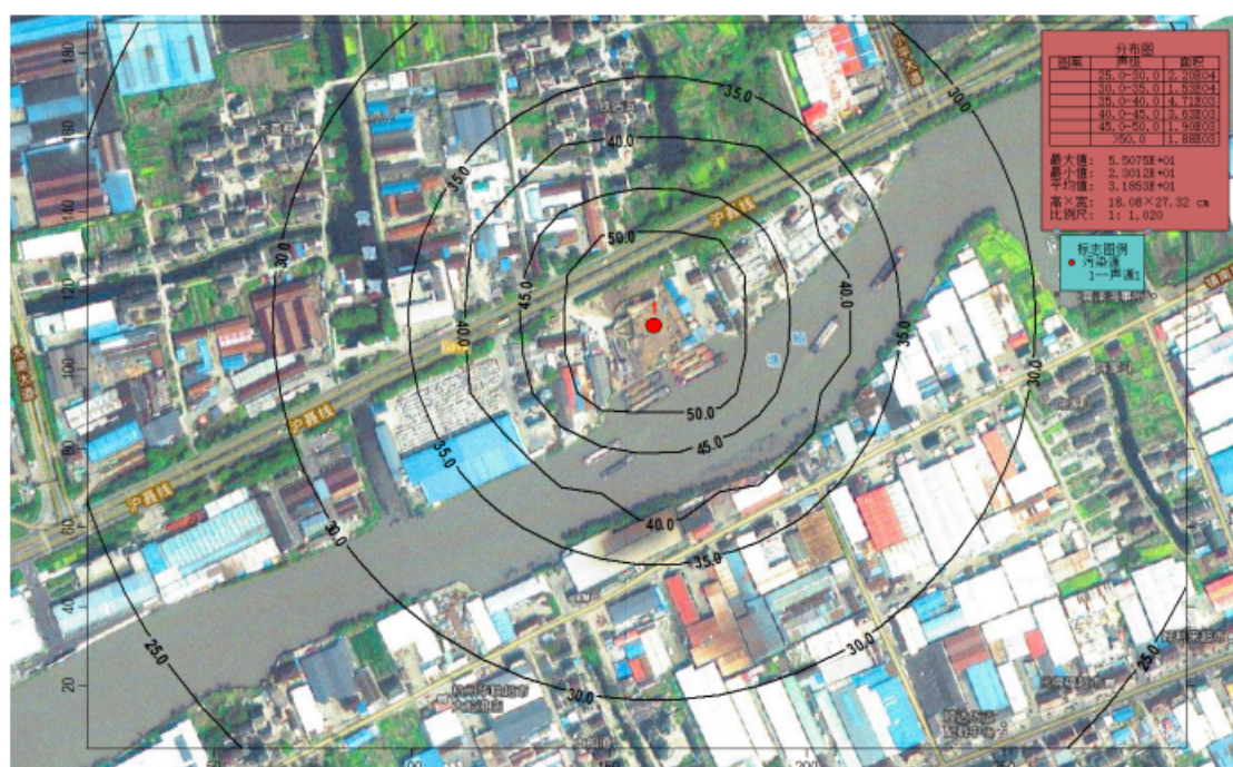
图 7-3 项目噪声预测等声级线图
