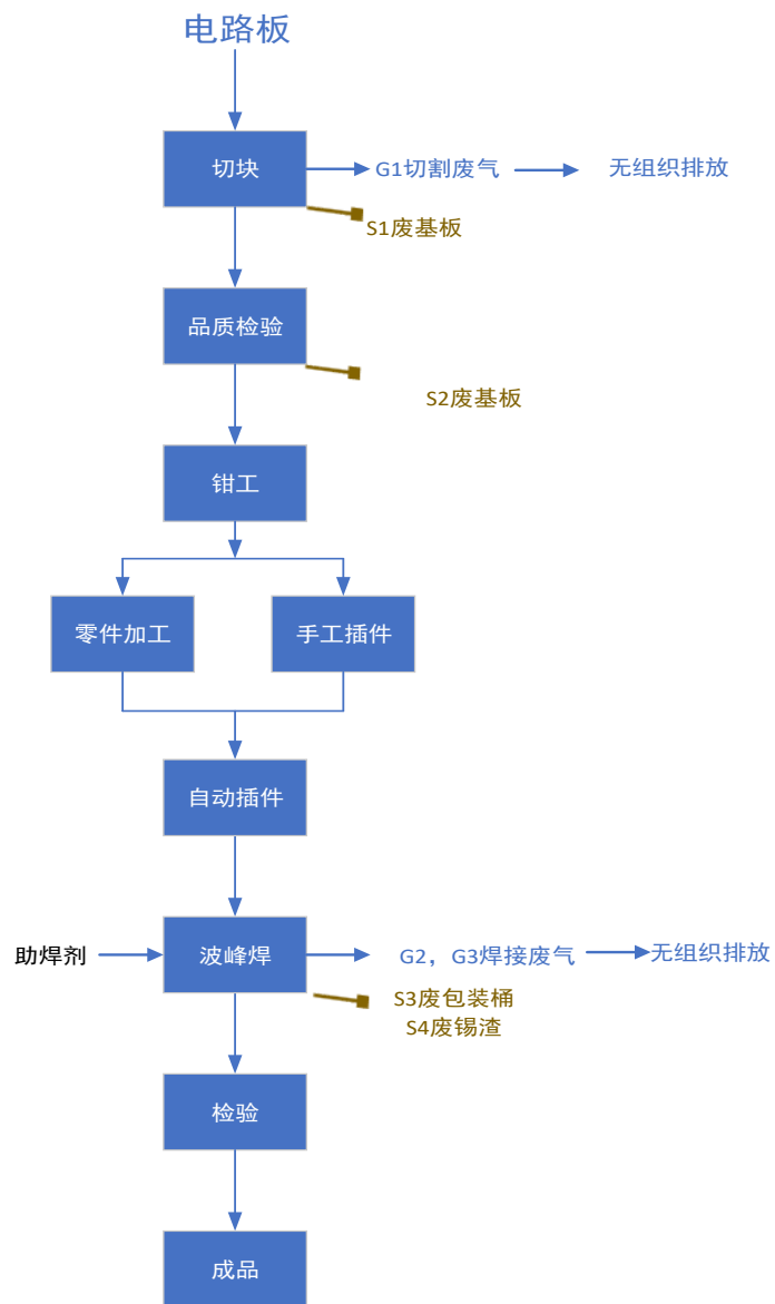
图 1-1 现有项目工艺流程图
