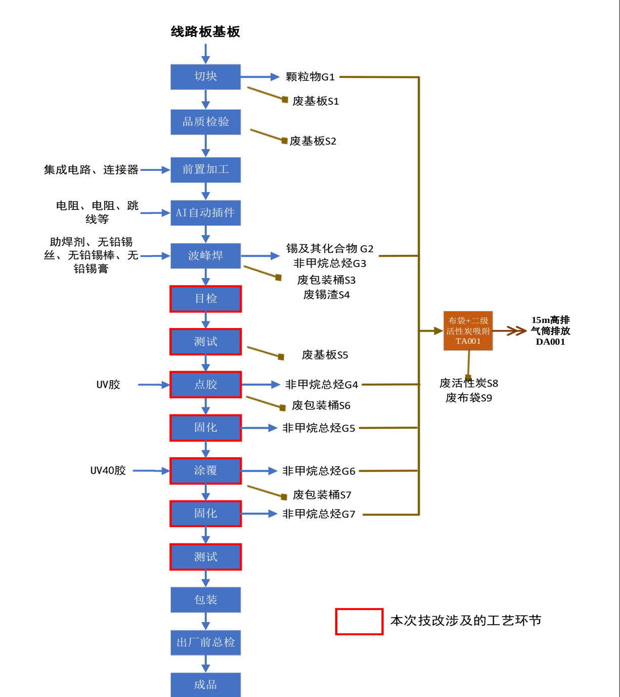
图 5-1 本项目工艺流程图
