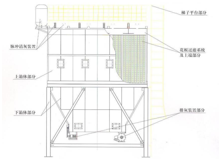
图 7-1 布袋除尘器原理图
