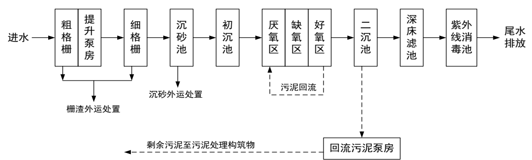
图 7-1 苏州市吴江经济技术开发区运东污水处理厂处理工艺
