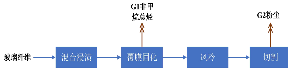
图 1-1 现有项目透明板生产工艺流程图
