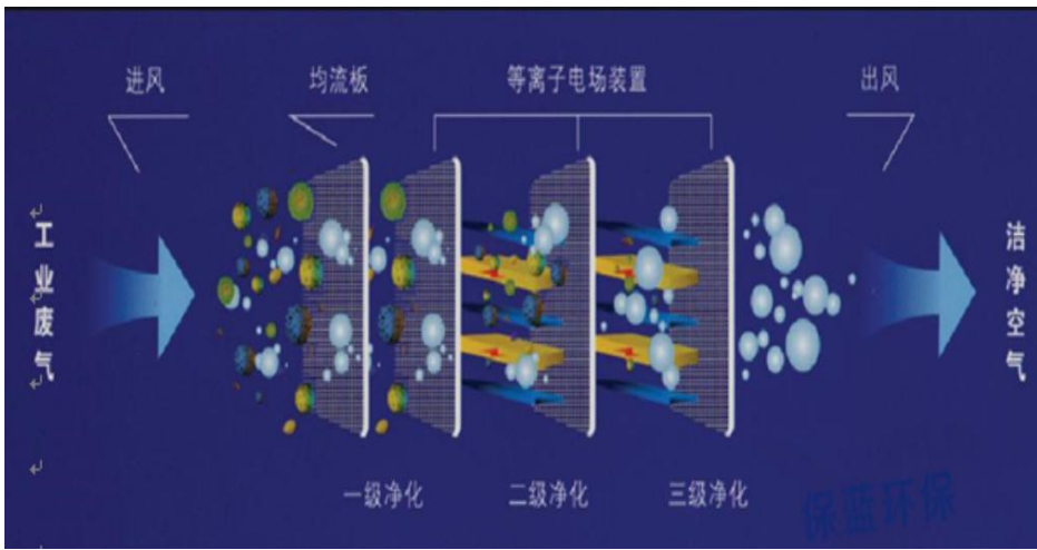
图 7-1 低温等离子原理图
