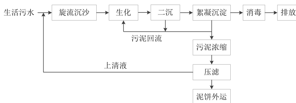
图 7-2 苏州市吴江震泽生活污水处理有限公司处理工艺
